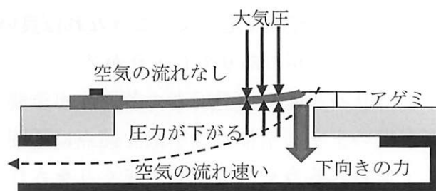
図3：息を吸い込んだ時
