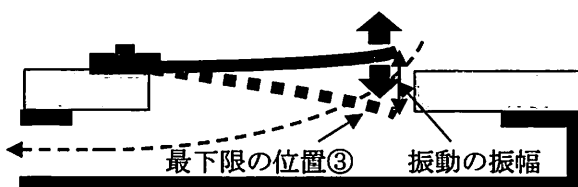
図6：リードが戻ったとき
