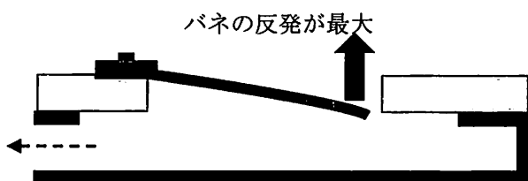
図5：リードが最下面に
