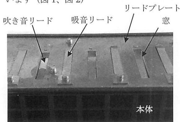
図1：リードプレート構造（複音）
