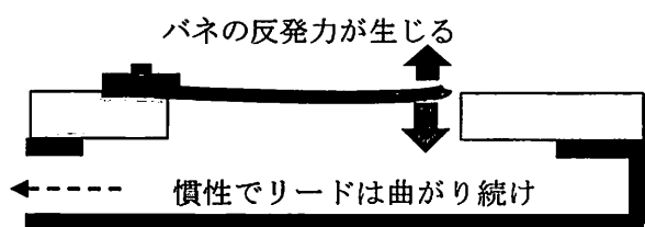
図4：リードがプレート面に達したとき
