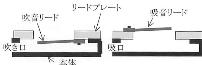
図2：ハーモニカ模式図
